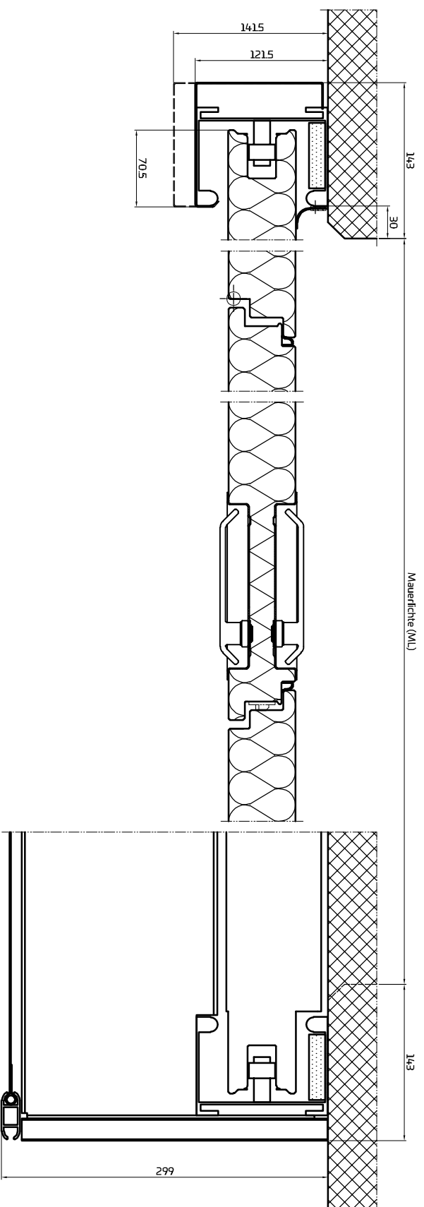
Seitenführung Hubtor mit Rauschschutz und eingebauter Fluchttür
